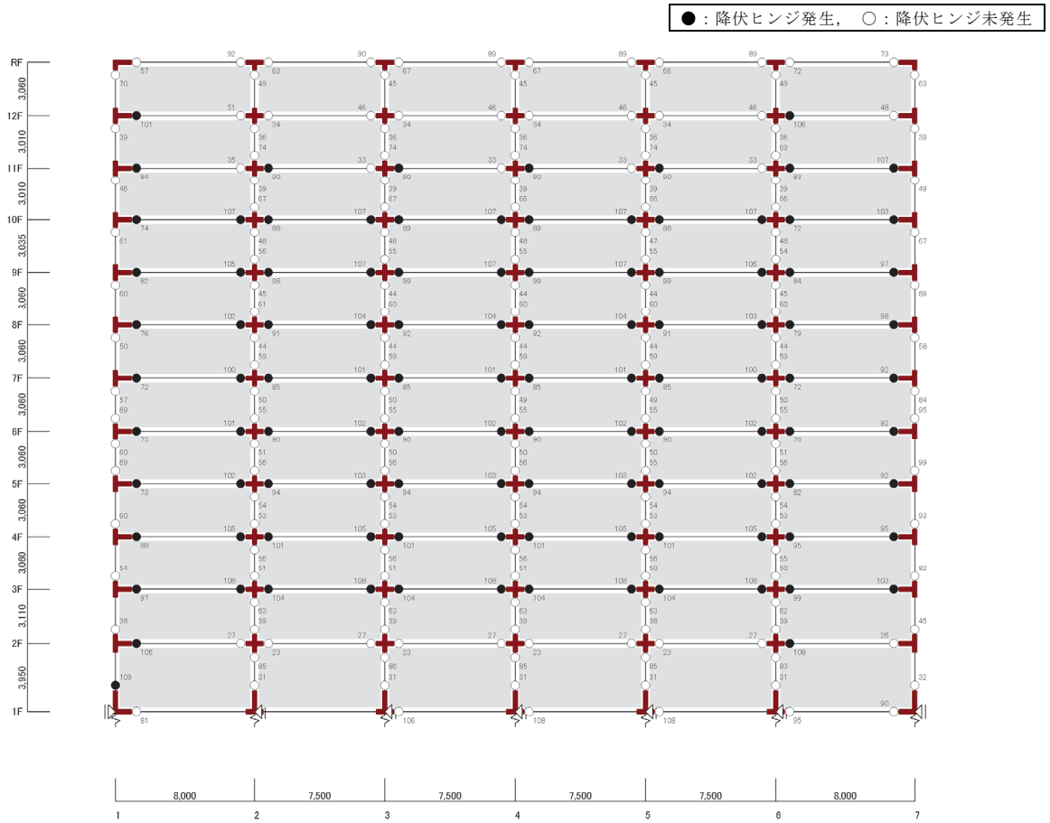
図 1.2 D s 算定時 A 通架構ヒンジ図(左加力)
