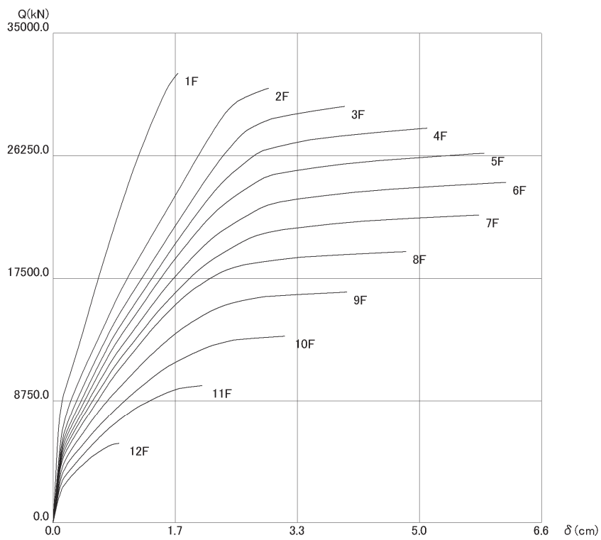
図 1.3 A 通架構の増分解析結果(左加力)
