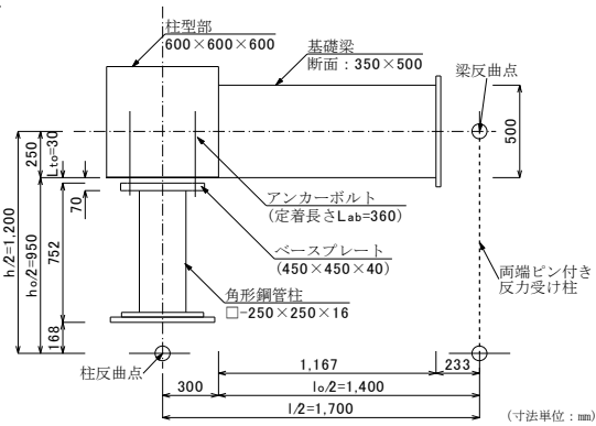
図 1 試験体全体寸法および加力方法 表 1 実験計画
