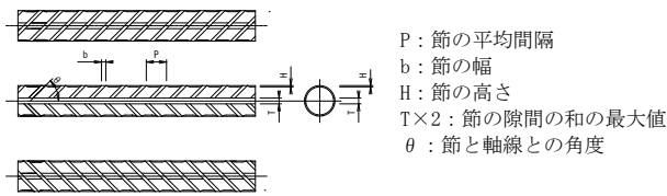
図 1 SPR685 の節形状
